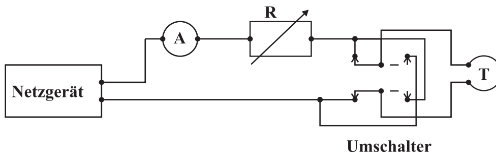
Abbildung 1: R = Regelbarer Widerstand, T = Tangentenbussole, A = Ampèremeter
